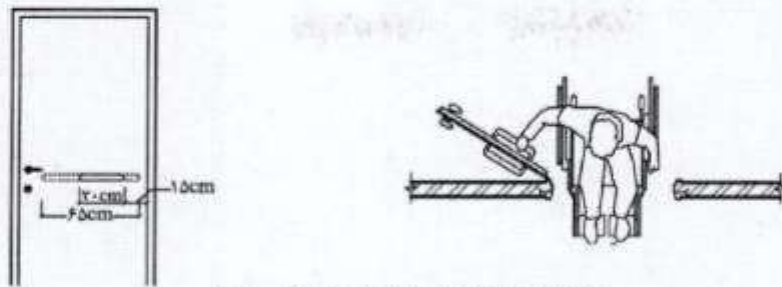
شکل شماره ۷۲: ابعاد میله دستگرد کمکی روی در
