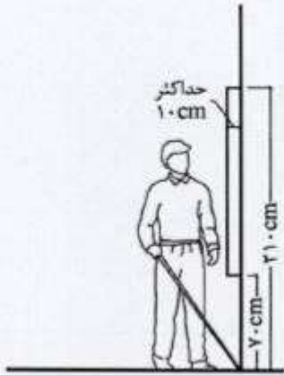
شکل شماره ۲۹: پیش‌آمدگی اشیای نصب شده روی دیوار در ارتفاع ۷۰ تا ۲۱۰ سانتیمتر
