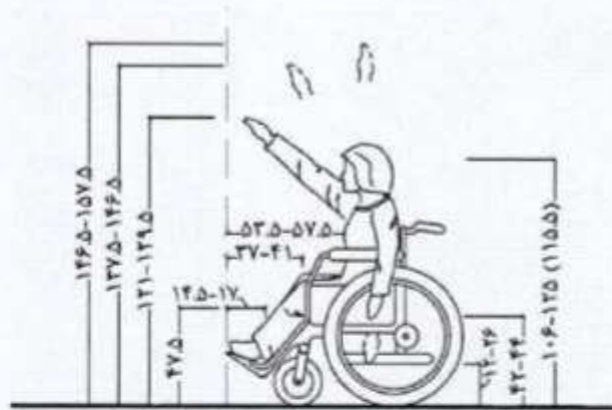
شکل شماره ۵: اندازه‌ها و دسترس‌های زن دارای معلولیت در حرکت به بالا
