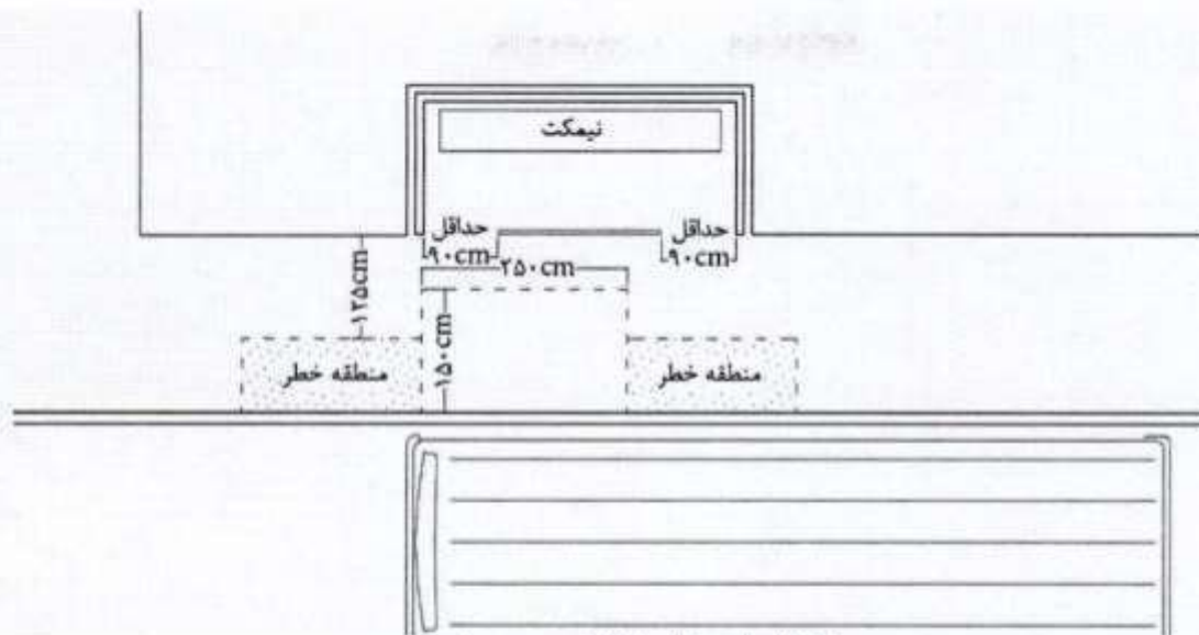
شکل شماره ۴۰: ایستگاه اتوبوس سرپوشیده
