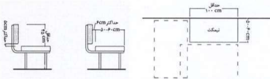
(ب) ارتفاع نشیمن و پشتی نیمکت
