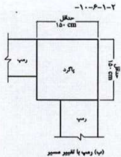
(ب) رسمب یا تغییر مسیر ۱-۲-۶-۱۱- شکل شماره ۶۱.
