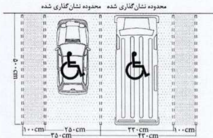
شکل شماره ۳۹: ابعاد فضا و مسیر دسترسی به محل توقف ویژه افراد دارای معلولیت
