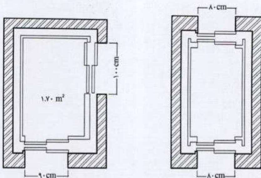
شکل شماره ۶۳: محل قرارگیری در آسانسور شکل شماره ۶۴: محل قرارگیری در آسانسور
