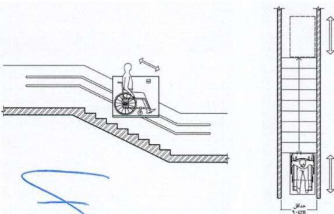
شکل شماره ۶۸: بالابر جانبی
