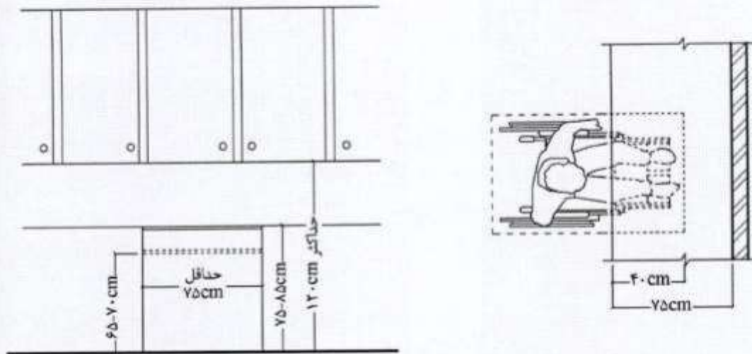
شکل شماره ۱۰۱: ابعاد دسترسی و فضای آزاد جلوی سطح کار جهت قرارگیری صندلی چرخدار
