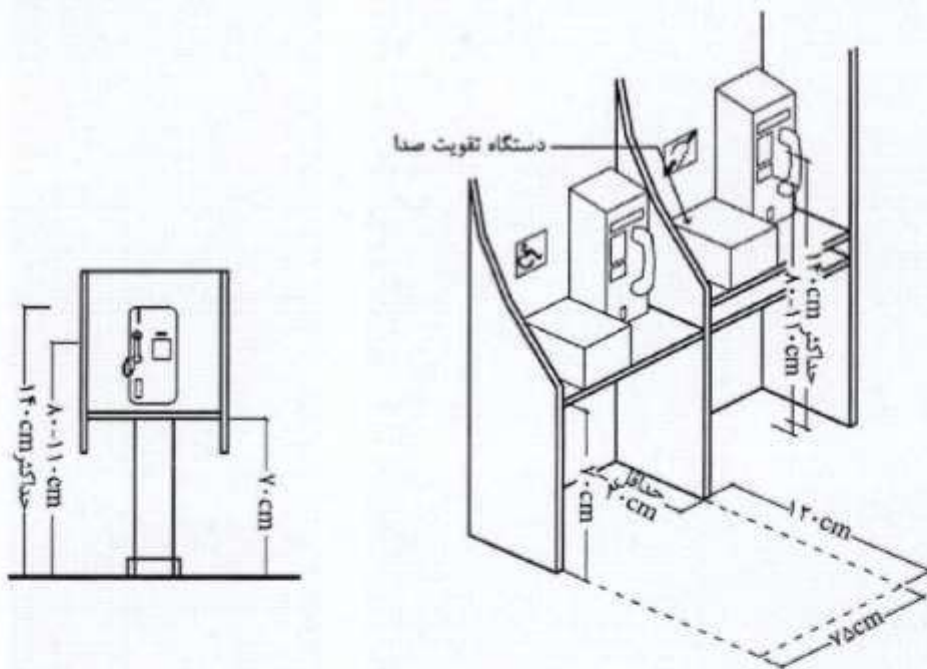
شکل شماره ۴۸: تلفن عمومی دسترس‌پذیر
