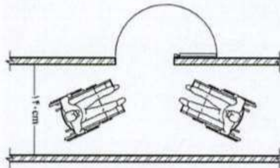
شکل شماره ۵۴: حداقل عرض راهرو
