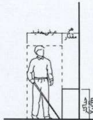
شکل شماره ۲۸: پیش‌آمدگی اشیای نصب شده روی دیوار تا ارتفاع ۷۰ سانتیمتر
