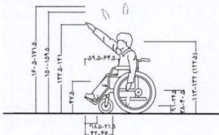
شکل شماره ۳: اندازه‌ها و دسترسی‌های مرد دارای معلولیت در حرکت به بالا
