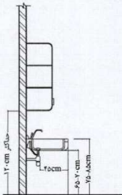
شکل شماره ۱۰۲: ابعاد و اندازه زیر سطح کار یا ظرفشویی جهت فرارگیری صندلی چرخدار
