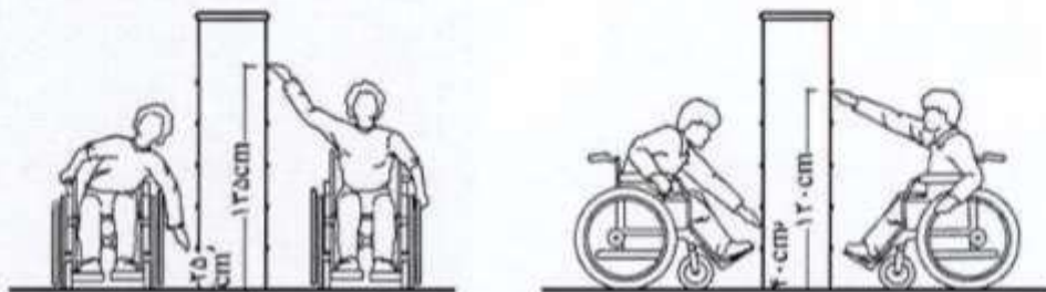
شکل شماره ۹۵، اندازه‌های مناسب برای دستیابی به قفسه‌ها از پهلو و مقابل
