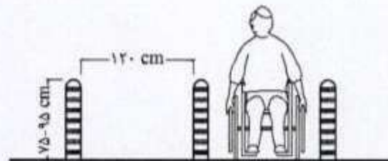
شکل شماره ۲۶: ابعاد و فاصله بین دو میله هدایت‌کننده
