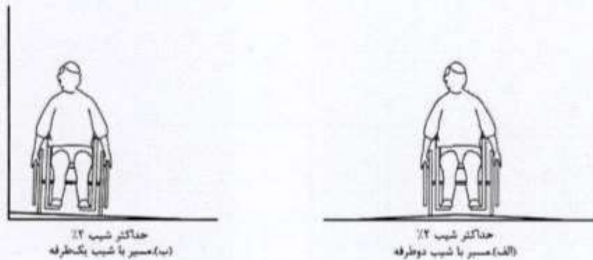
شکل شماره ۲۵: حداکثر شیب عرضی پیاده‌رو
