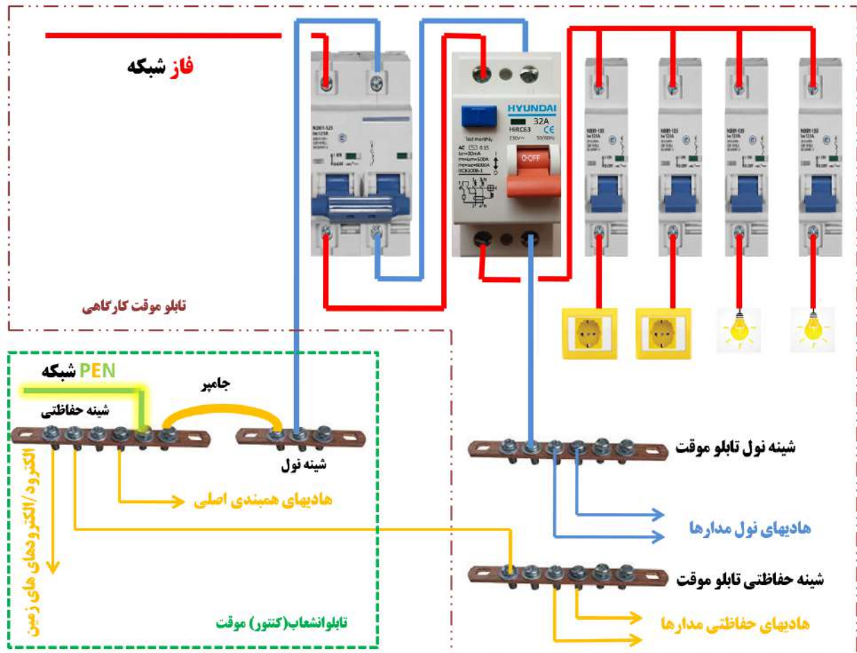
نمونه تابلوی موقت کارگاهی و انشعاب موقت (تک فاز) (با رعایت الزامات سیستم نیروی TNCS)
