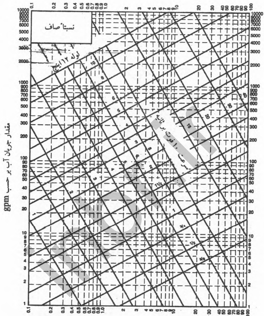
افشار آب بر حسب پوند بر اینچ مربع در ۱۰۰ فوت طول
