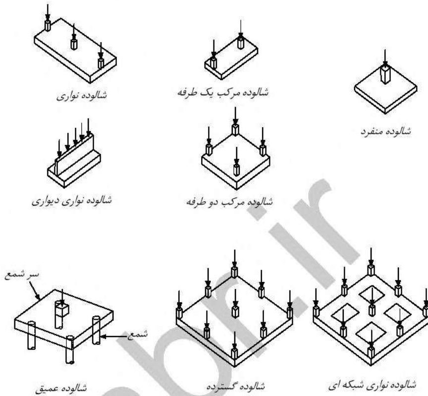
شکل ۹-۱۵-۱ انواع شالوده‌ها
