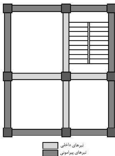
شکل ۹-۶-۱ تیرهای داخلی و پیرامونی
