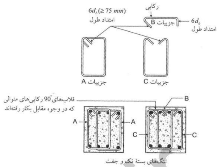
شکل ۹-۶-۴ جزئیات اجرایی دورگیرها
