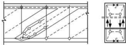
ب- عضو فشاری قطری در جان دارای خاموت
