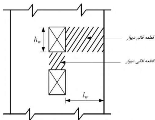
شکل ۱-۲۰-۹ دیوار سازه‌ای با باز شو
