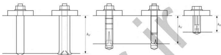
مهار انبساطی علاف‌دار
