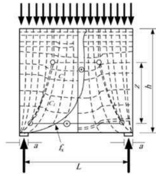
ب- میدان تنش و مدل خرابایی برای یک تیر تیرغه
